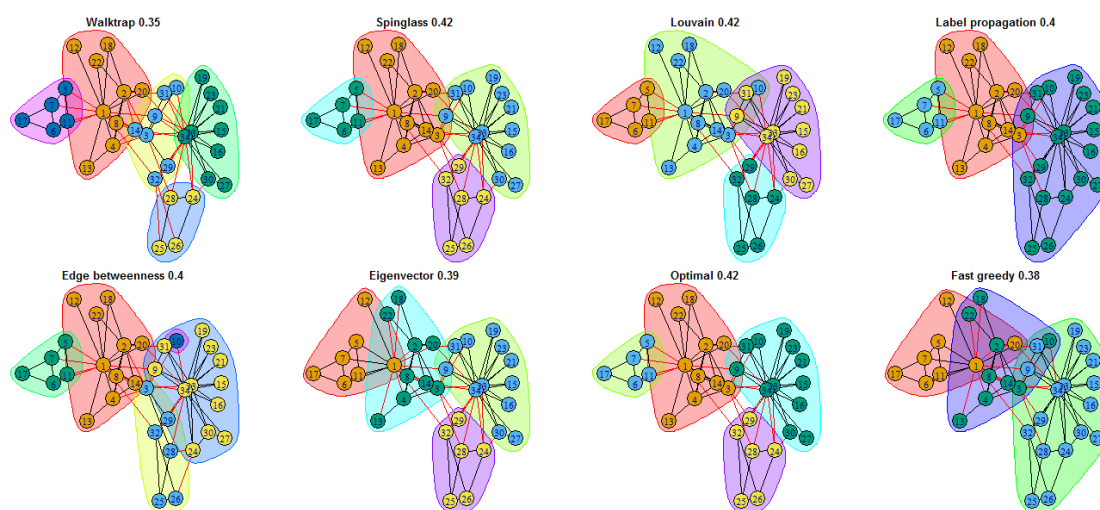
FIGURE 6.4 – Un réseau, x méthodes de détection de communautés
