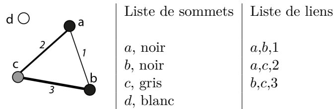
FIGURE 4.1 – Graphe, liste de liens, matrice d'adjacence
