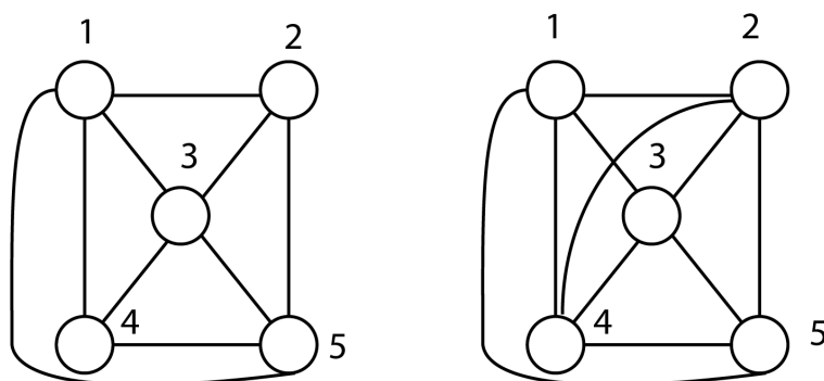
Le réseau de gauche est planaire, aucune arête ne se croise. Il est également complet ; le seul lien manquant (2-4) ne peut être ajouté sans provoquer une intersection de liens. Le réseau de droite est non planaire et complet.
